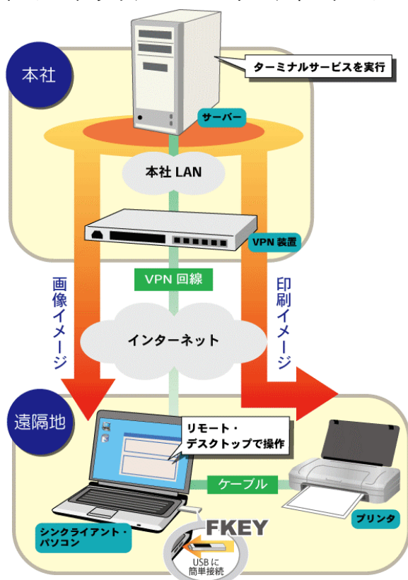
図：シンククライアント・プリンティング・システム
